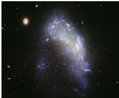
NGC 1427A
