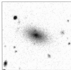
Fig. 1 g: FCC #195
