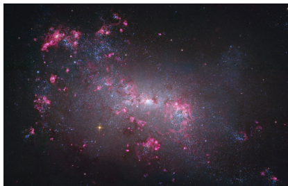
NGC 4449
